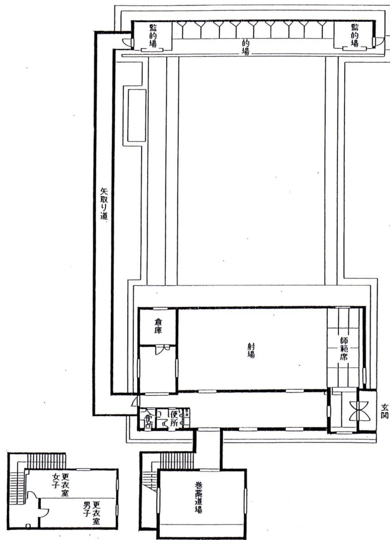
2階平面図
